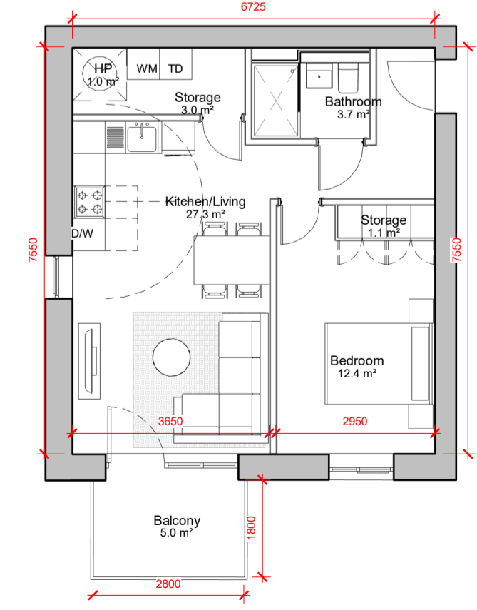
6 1 BED TYPE P 1 : 100
