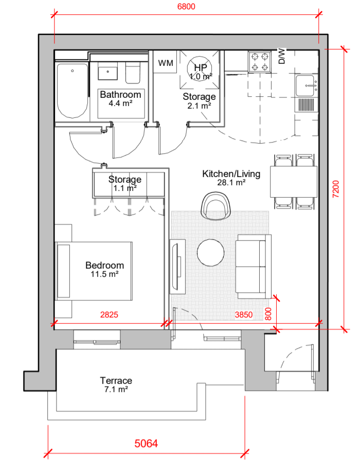
4 1 BED TYPE N 1 : 100
