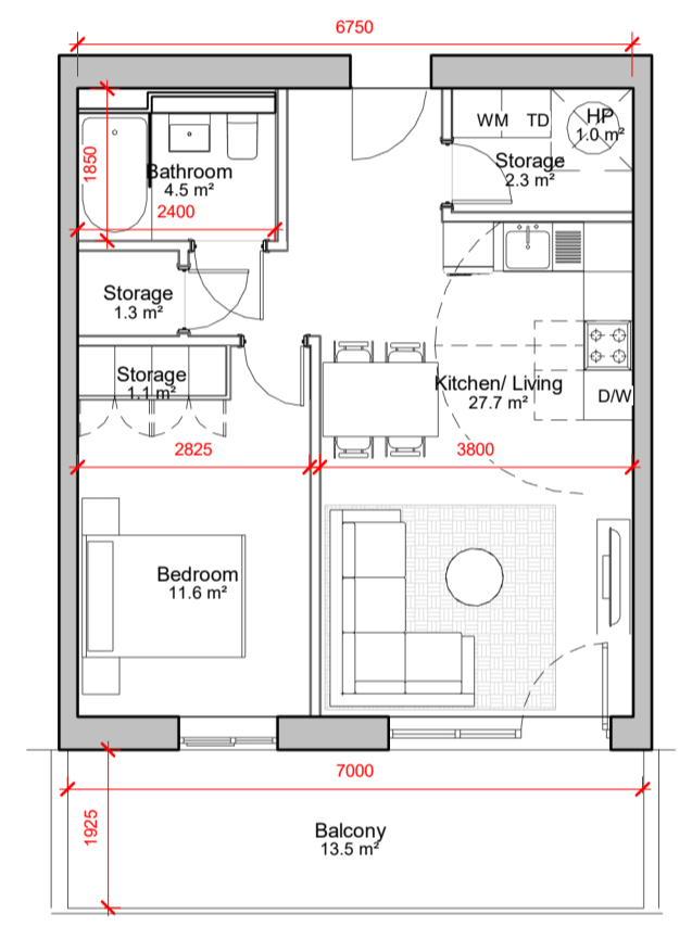
5 1 BED TYPE O 1 : 100
