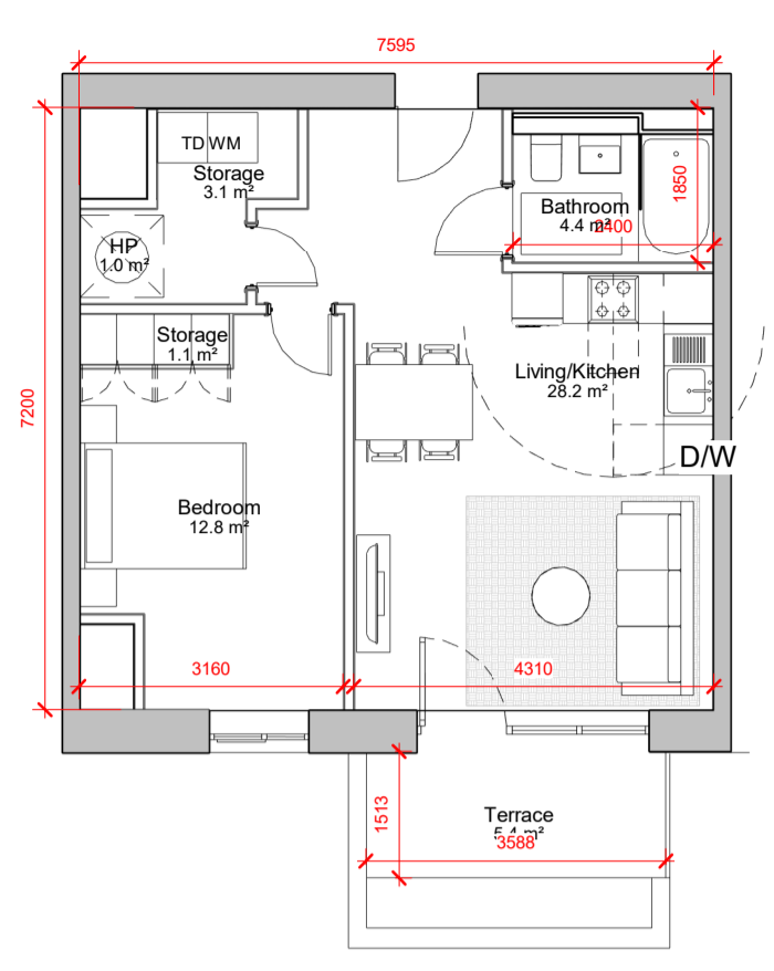
10 1 BED TYPE M 1 : 100
