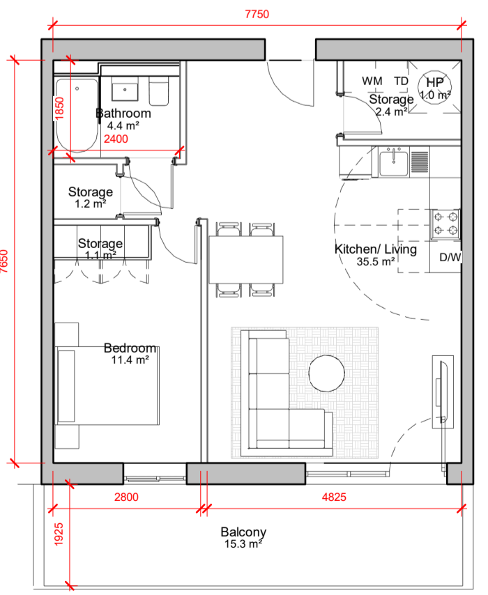
3 1 BED TYPE O2 1 : 100
