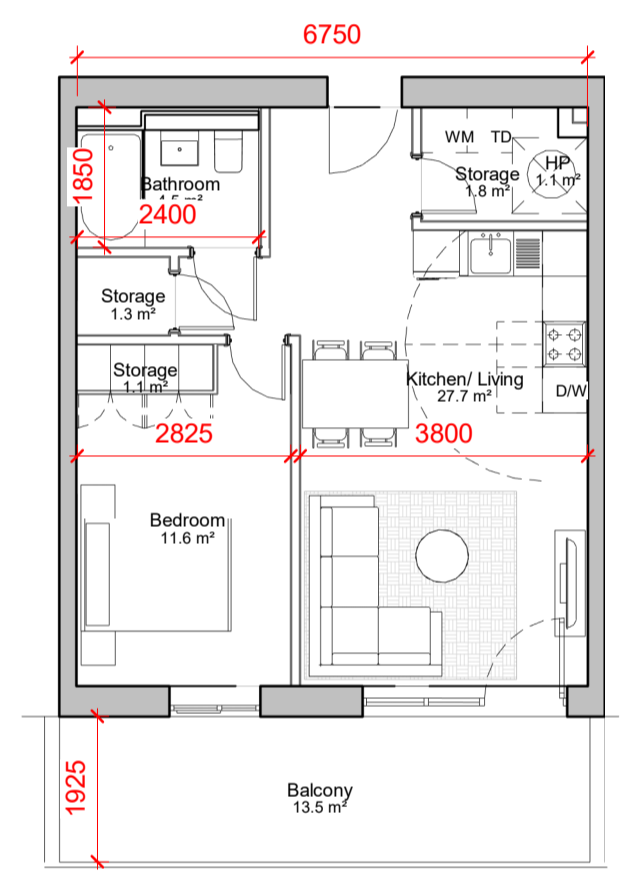
8 1 BED TYPE O3 1 : 100
