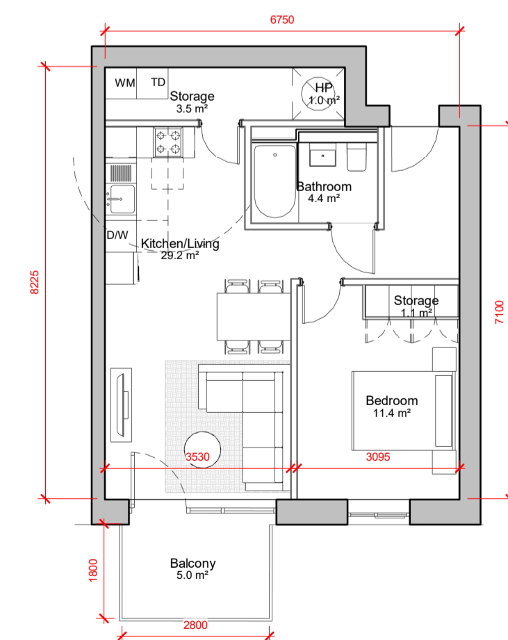
7 1 BED TYPE Q 1 : 100
