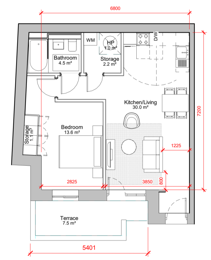
2 1 BED TYPE N2 1 : 100
